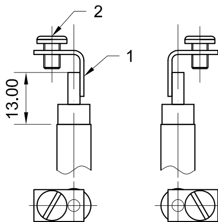
PROVEDENÍ 4 15A - Ø6,5 16A - Ø8,5
