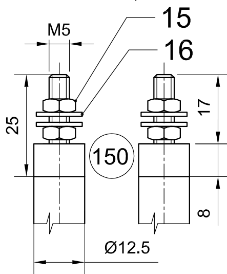
40A (Ø 12,5)
