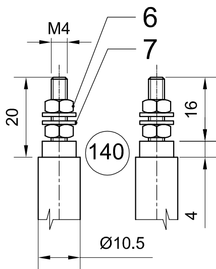
25A (Ø 10,5)
